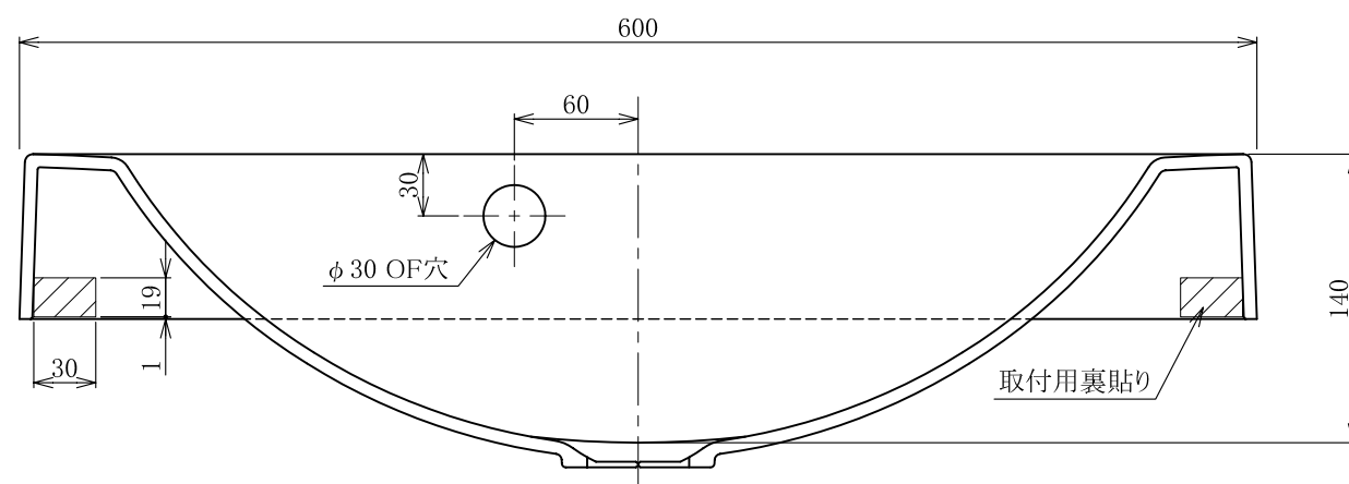
A-A 断面図
